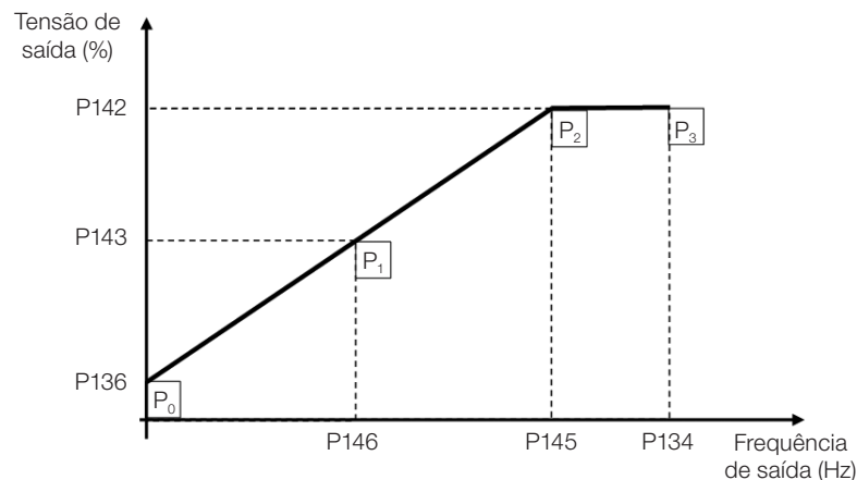
Figura 9.2: Curva V/f
