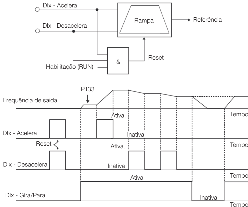
Figura 7.4: Gráfico de funcionamento da função E.P.
