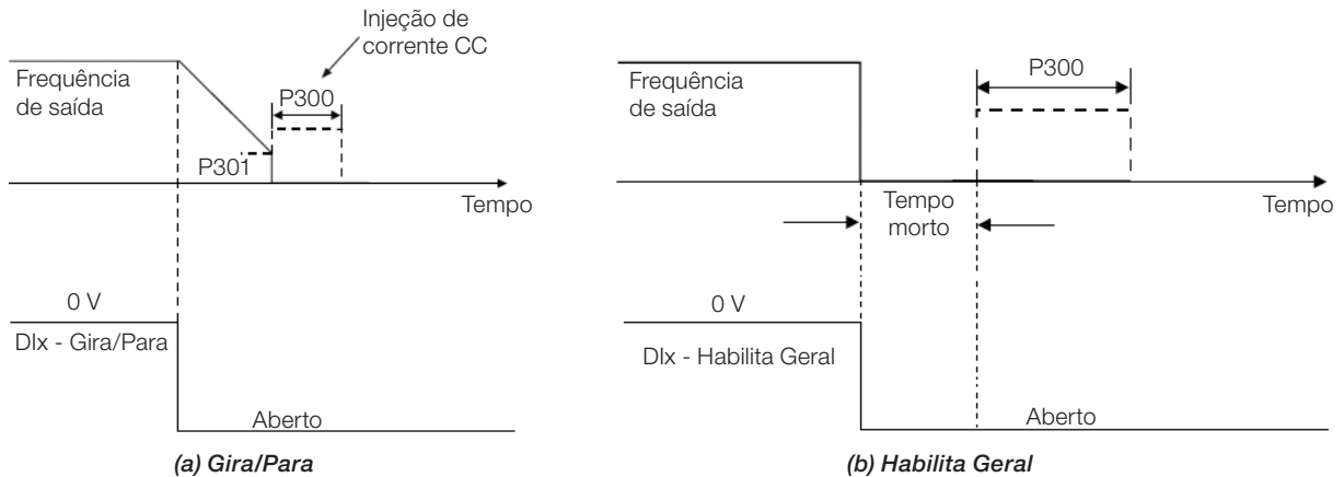
Figura 11.8: (a) e (b) Atuação da frenagem CC na parada com comando
