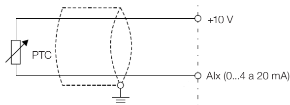
Figura 14.2: Conexão do PTC ao CFW300
