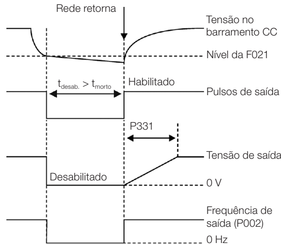
Figura 11.6: Atuação da função Ride Through
